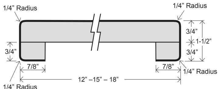
BAR TOP CNB 12 CNB 15 CNB 18
